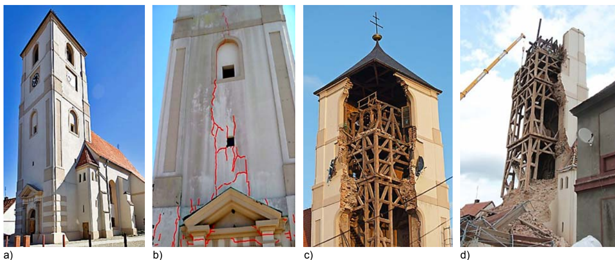
Ryc. 2. Widok kościoła w Otyniu, a) przed katastrofą (fot. T. Zuk), b) przed katastrofą (fot. PINB), c) w trakcie i d) po katastrofie (fot. www.parafia-otyń.pl )
