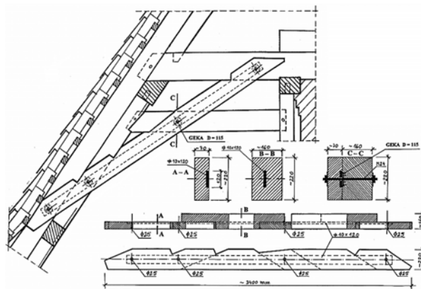
Ryc. 26. Koncepcja wzmocnienia zastrzału za pomocą wklejonego w drewno płaskownika stalowego
